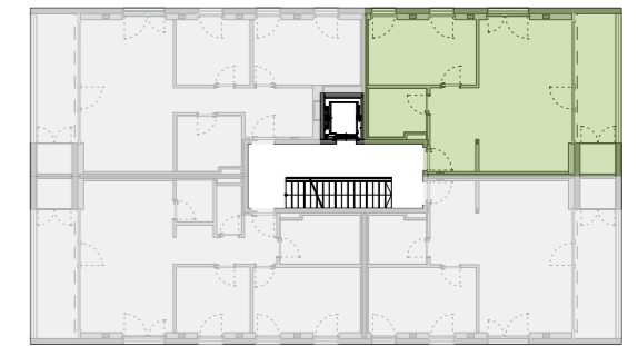
Übersicht 1.OG
