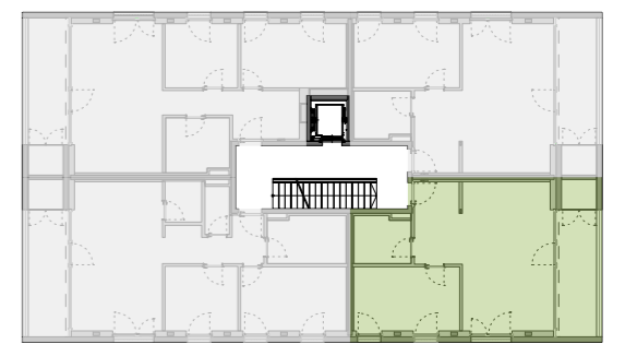
Übersicht 1.OG
