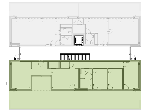
Übersicht EG
